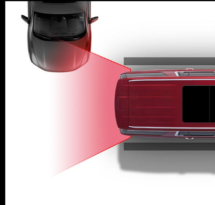
ALERTA DE TRÁFICO TRASERO CRUZADO
